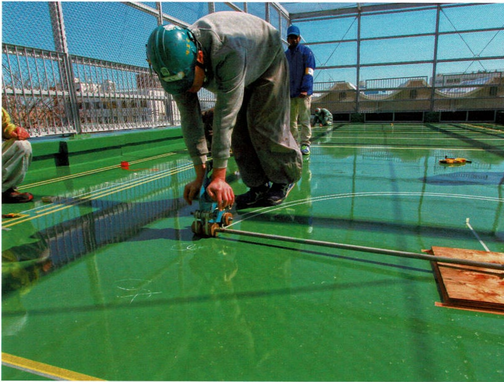
小径サークルラインのマス킹作業
